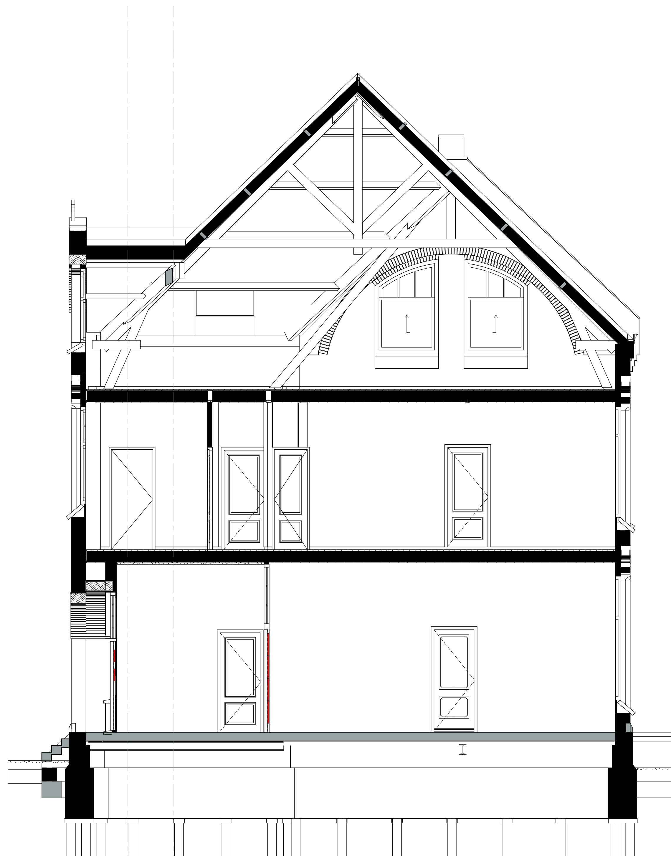
Doorsnede A5-A5
