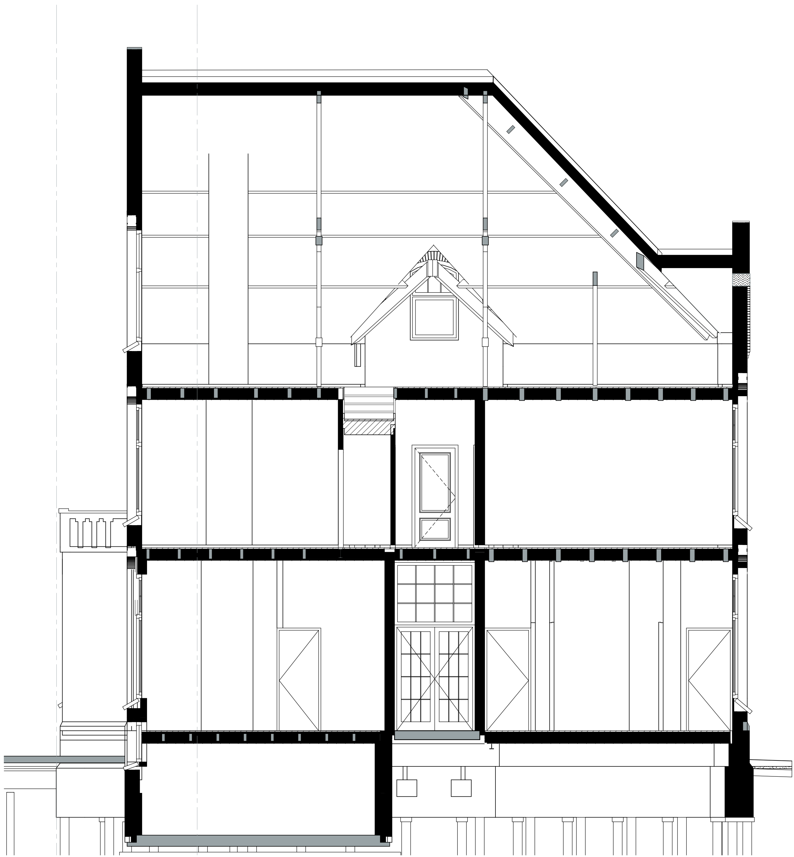
Doorsnede B-B
