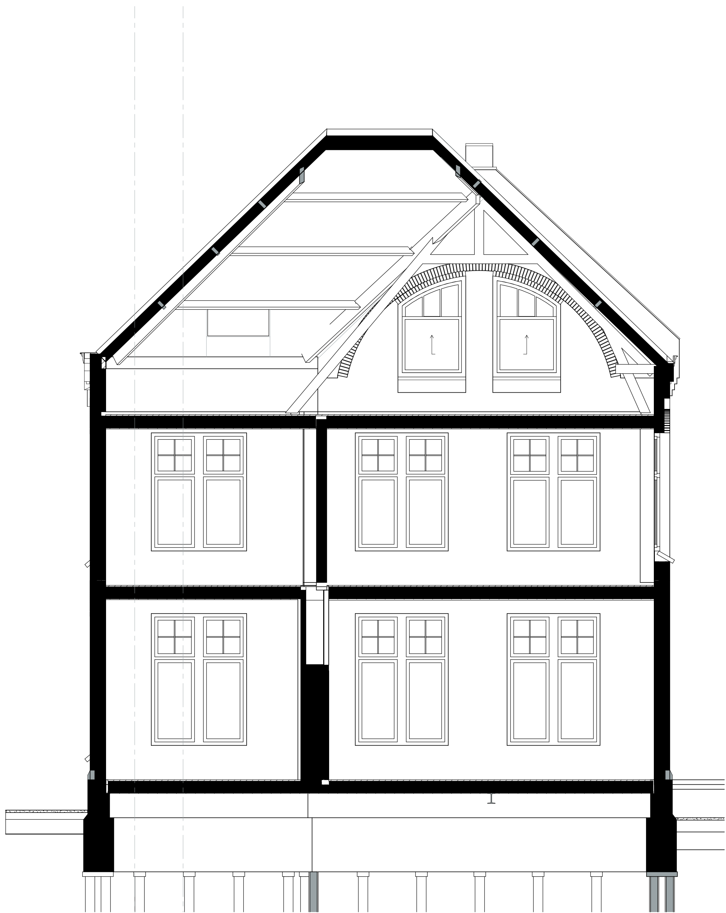
Doorsnede A4-A4
