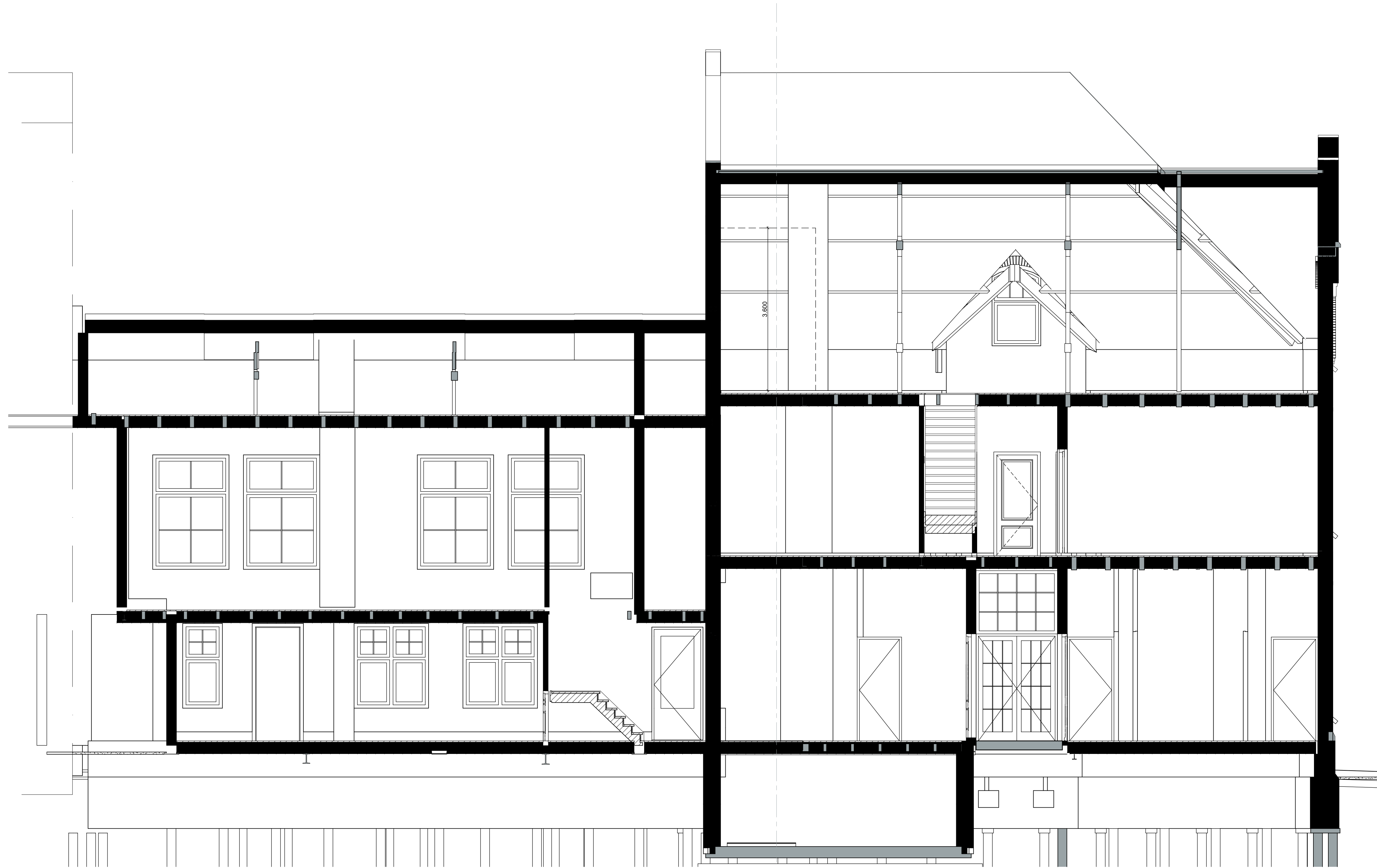
Doorsnede B1-B1
