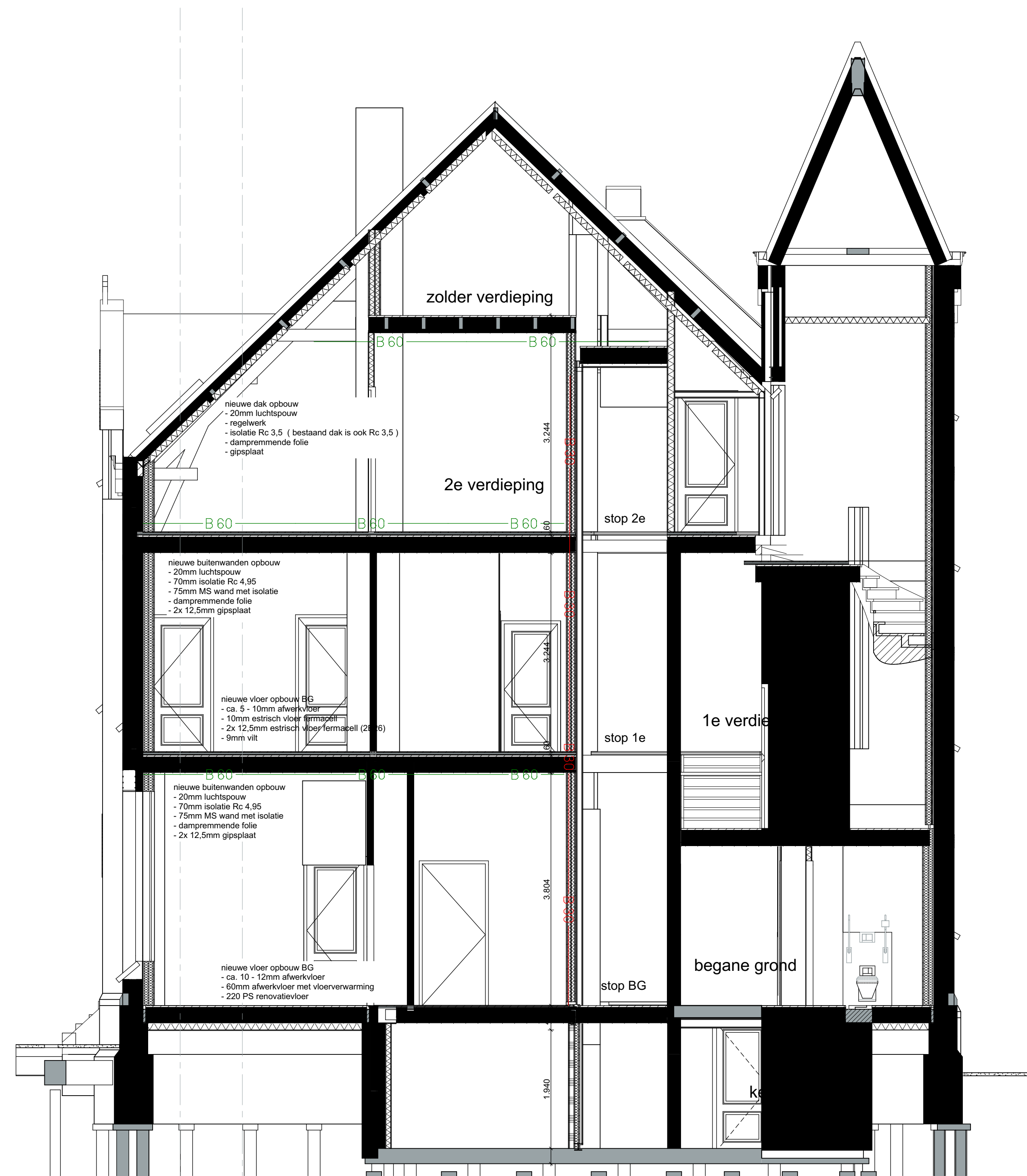
Doorsnede A6-A6
