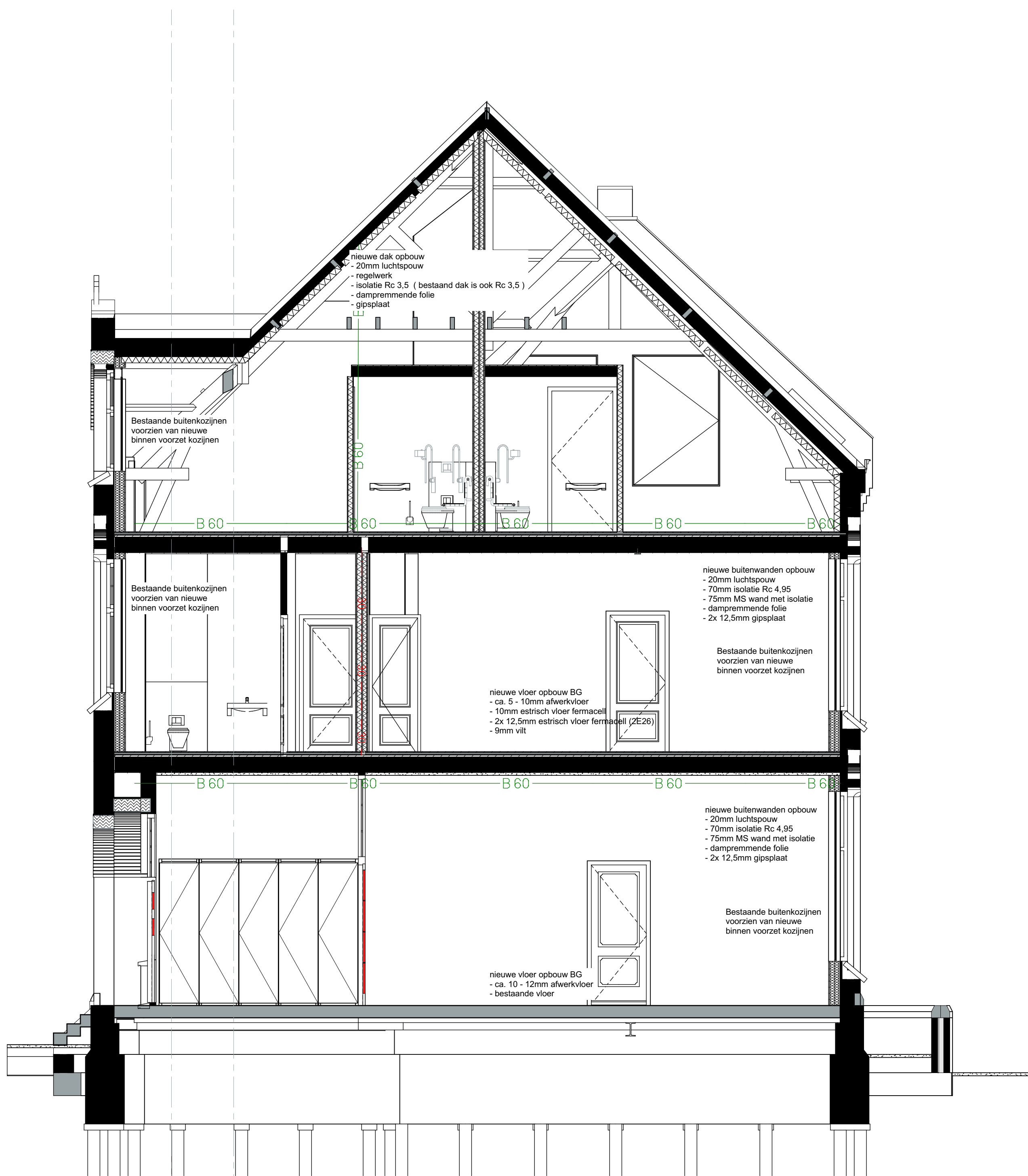
Doorsnede A5-A5
