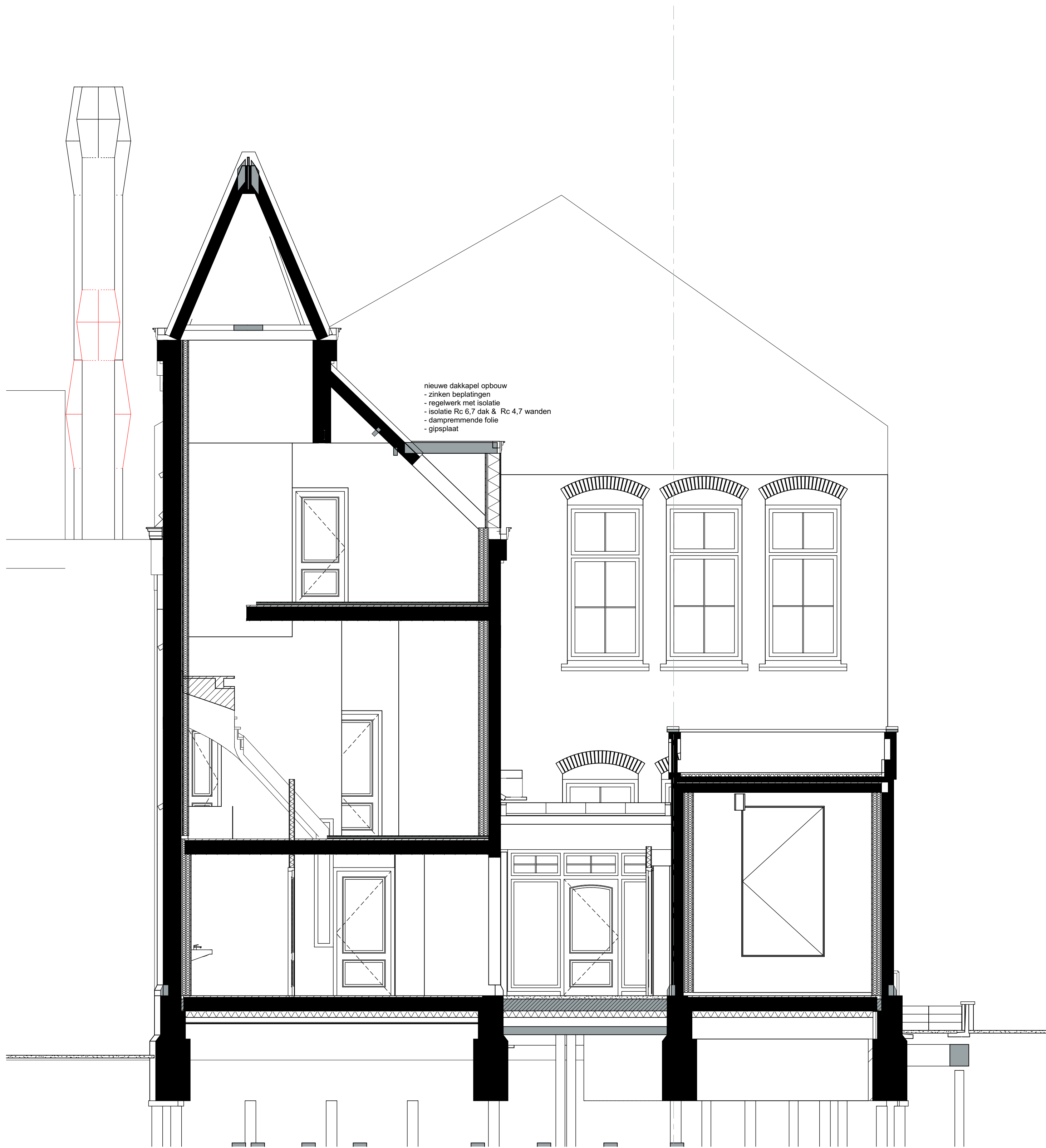
Doorsnede A3-A3
