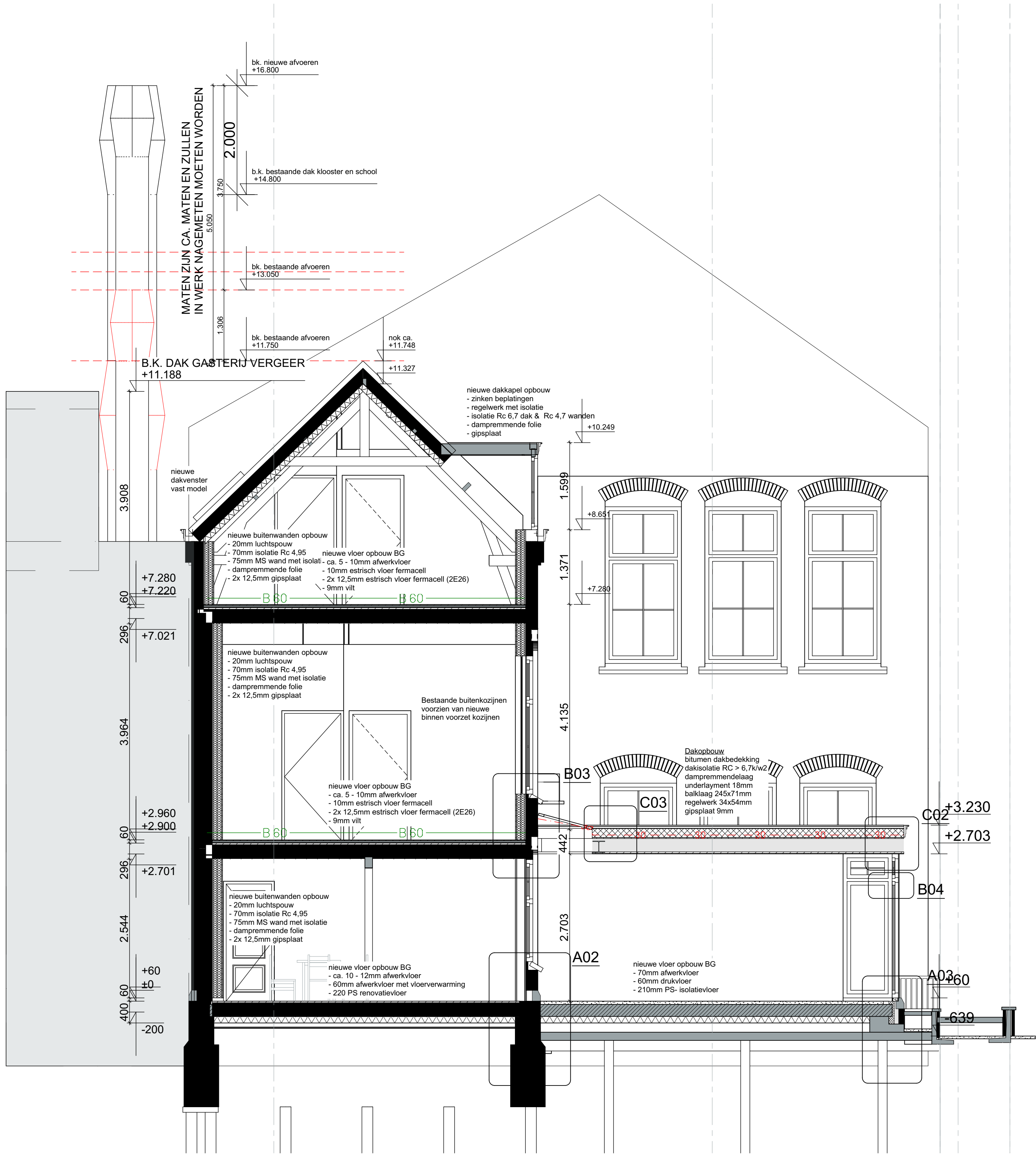
Doorsnede A2-A2
