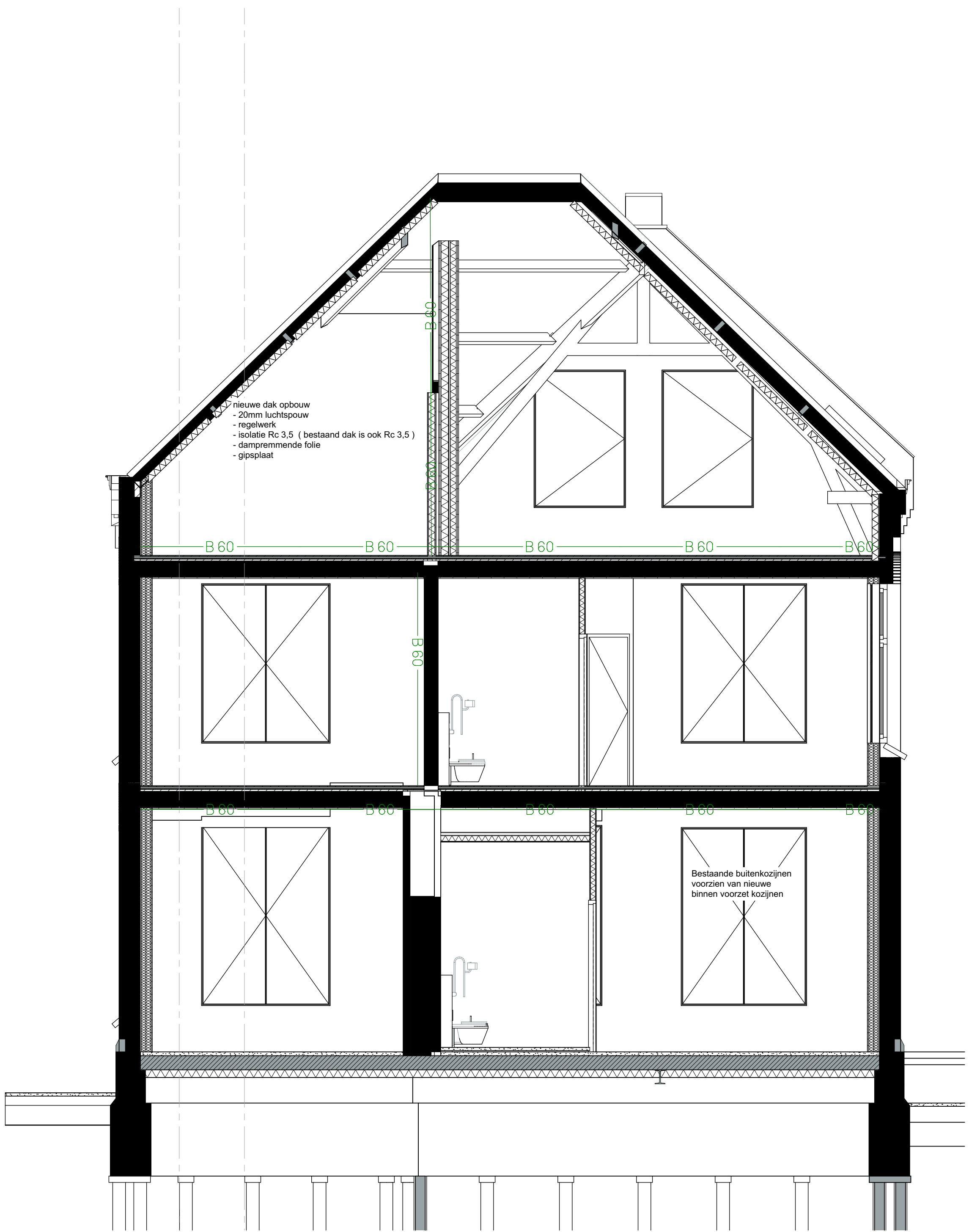
Doorsnede A4-A4
