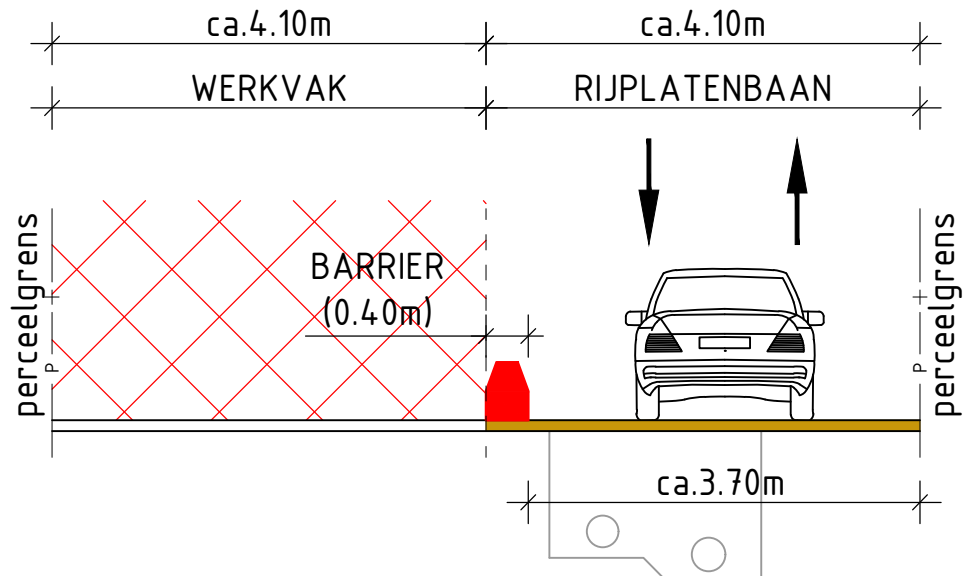
FASE 4B: WERKVAK / OM&OM-REGELING
