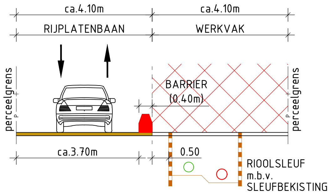
FASE 4A: WERKVAK / OM&OM-REGELING
