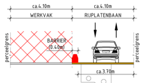
FASE 4B: WERKVAK / OM&OM-REGELING
