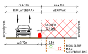
FASE 4A: WERKVAK / OM&OM-REGELING
