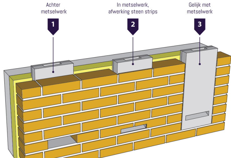
Figuur 12: Mogelijkheden plaatsing van vleermuiskasten in een gevel
