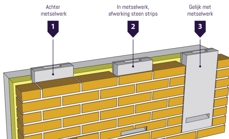
Figuur 17 Mogelijkheden plaatsing van vleermuiskasten in een gevel
