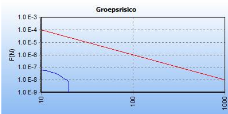
5.2 Figuur 5.2 FN curve voor 7584_leiding-W-501-04-deel-1 van N.V. Nederlandse Gasunie voor de kilometer tussen stationing 0.00 en stationing 150.00
