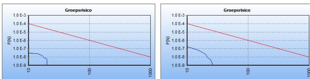
Figuur 10. Groepsrisico W-501-12, huidig (links) en toekomstig (rechts)
