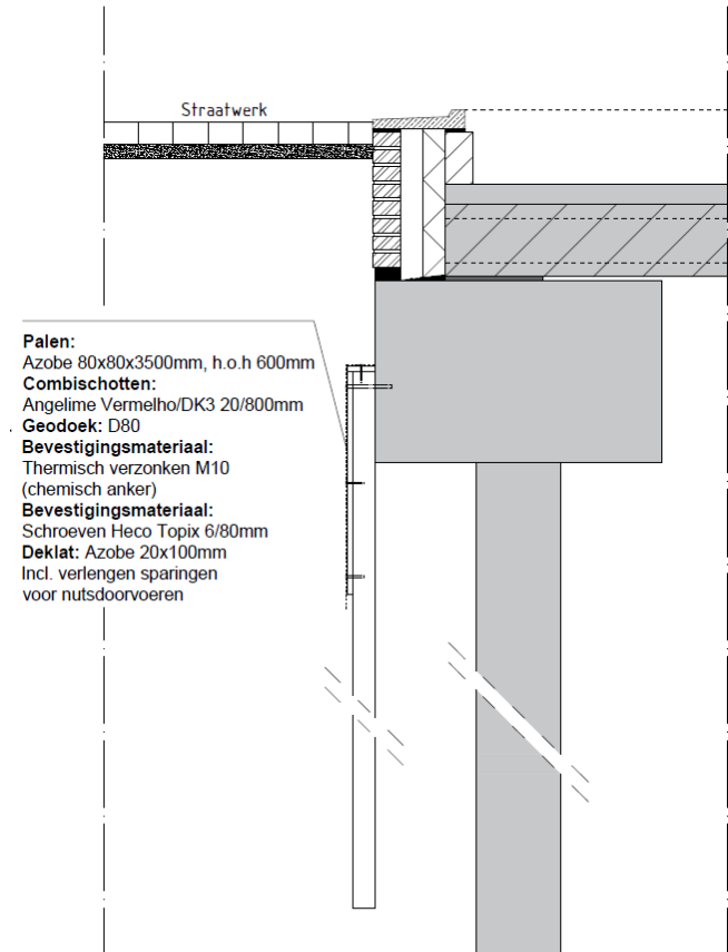
Principedetail onderspoelingsconstructie (1:10) Variant C
